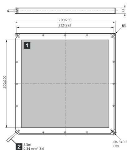
2) Anschlusskabel
