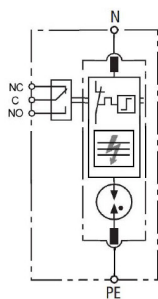
N-PE (GDT module)
