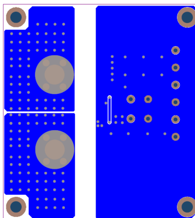
Bottom Layer
