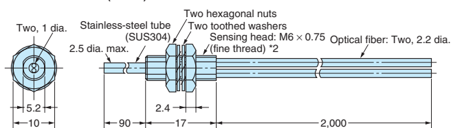
E32-DC200B(B4) E32-DC200BR(B4R)
