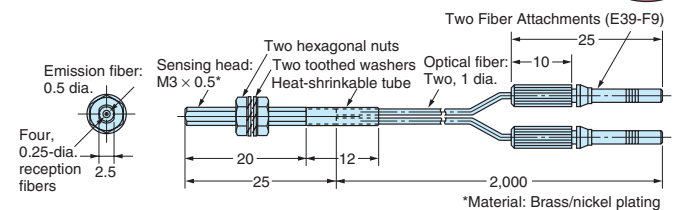
E32-C31
