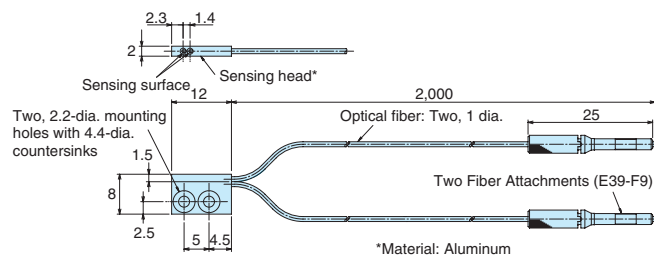
E32-D25Z E32-D25Z
