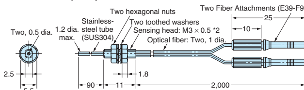
E32-DC200F(F4) E32-DC200FR(F4R)
