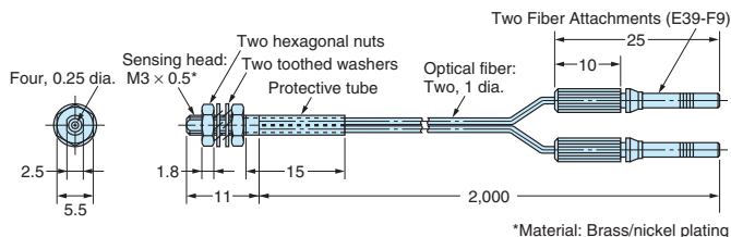
E32-D22B
