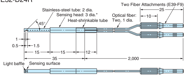
E32-D24 E32-D24R
