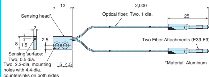
E32-DC200F(F4) E32-DC200FR(F4R)
