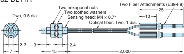
E32-D211 E32-D211R
