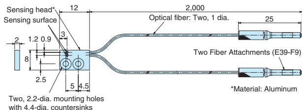
E32-D25Z E32-D25Z
