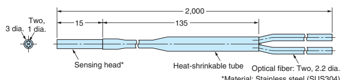
E32-D15X E32-D15XR
