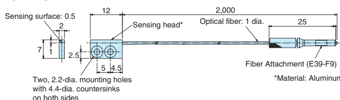
E32-TC200(F4) E32-TC200F(F4R)
