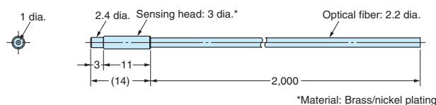
E32-T15X E32-T15XR
