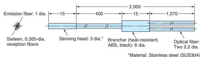
E32-D32L
