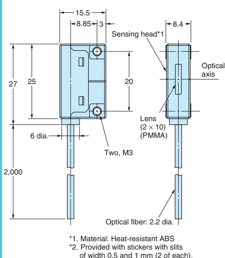
E32-T16
