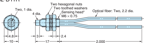
E32-DC200 E32-D11R
