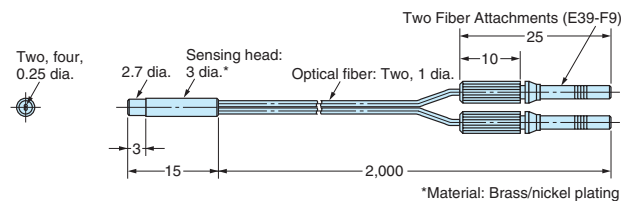
E32-D221B
