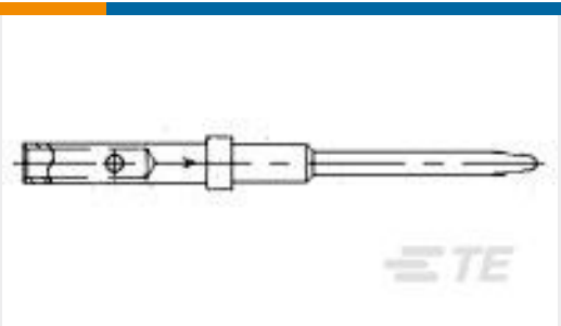
TE Part # 208262-3 5009-328-0022
