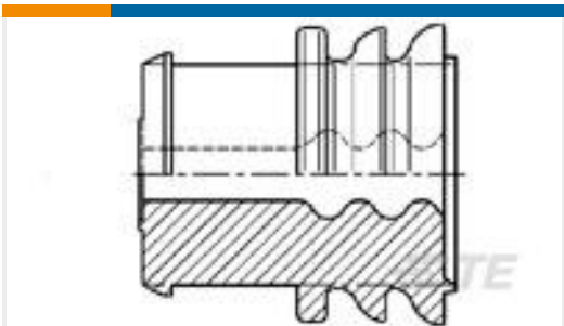
TE Part # 963245-1 EINZELLEIT-DICHTUNG
