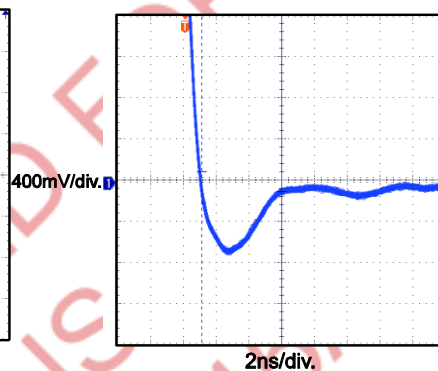
SW Falling Edge Dead Time
