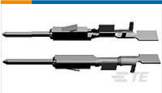
TE Part # 1355719-1 MQS0,63 Sn tab LL unseal. 0,08-0,22
