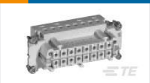
TE Part # 1-1103639-1 HE.16.BU.S.B 1-16
