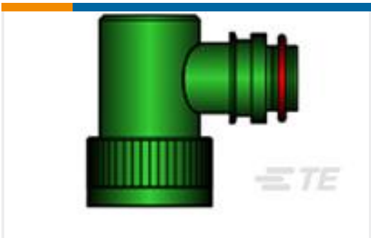
TE Part # 367328-000 TXR40AC90-2016AI
