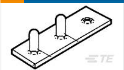
TE Part # 60843-1 2P CMNL COMM TAB PTPBR
