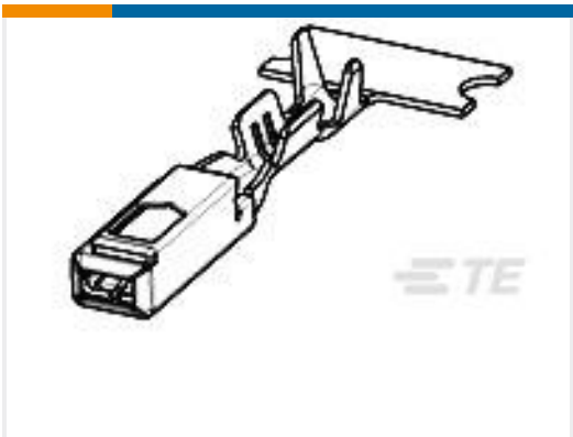
TE Part # 5-1534116-1 MQS0,63 SN REC CB UNSEAL. 0,25-0,35 2P
