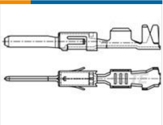
TE Part # 963898-1 MICRO TIM ST1,6X0,6
