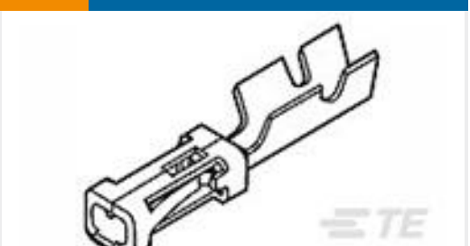
TE Part # 2-87523-3 MOD IV RECP PLTD 15 DPLX
