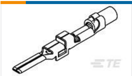
TE Part # 368087-1 090II NON SLD TAB(SQ0.85-1.25)
