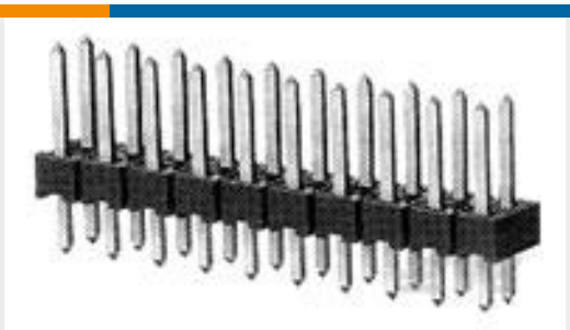
TE Part # 1-826656-0 10P AMPMODU II STIFT LEI
