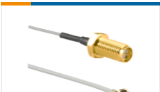
TE Part # CSI-RGFB-300-UFFR RP-SMA to U.FL/MHF1 300mm 1.13 OD
