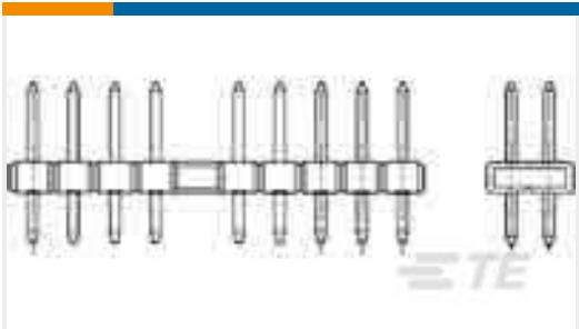
TE Part # 4-5176264-5 44 AMPMODU 2MM DR VERT MNT LF
