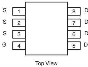
SO-8
