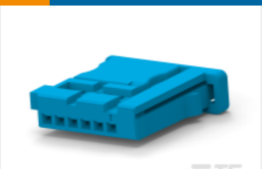
TE Part # 2282154-3 6POS,NANOMQS,REC HSG,CODC
