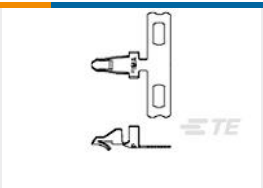
TE Part # 350566-3 MINI AMP-IN 22-18 PTPBR
