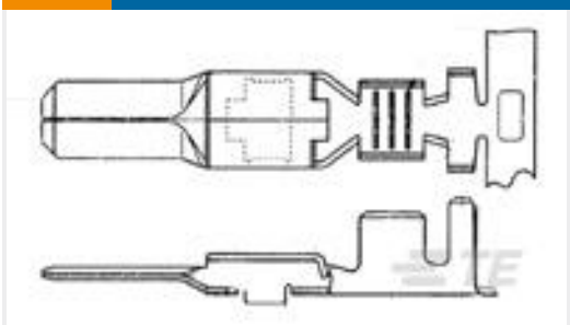
TE Part # 175048-1 FF 187 TAB 2-3MM2 PTBR
