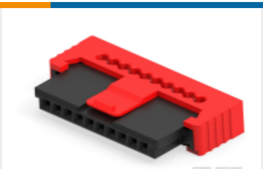
TE Part # 234465-E SRCP 1,27 10 F 1 I2426 137 E1 162 1,07 T
