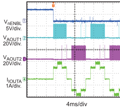
Enable-Half Step
