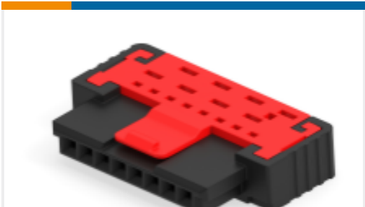
TE Part # 214159-E SRCA 1,27 8 F 1 I2426 137 E1 094 1,07 TR
