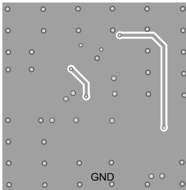
Bottom Layer
