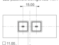
LED Platzierung mit Leuchtfeld 11x11 LED placement with light field 11x11
