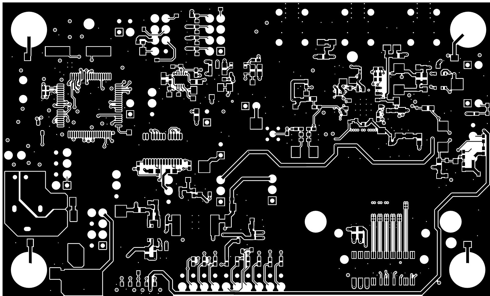
Figure 16-9. Layer 8: Bottom Signal Layer
