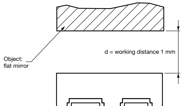
Fig. 3 - Test Setup
