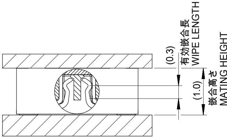
嵌合断面図 ( 参考 ) MATED DRAWING (REFERENCE)
