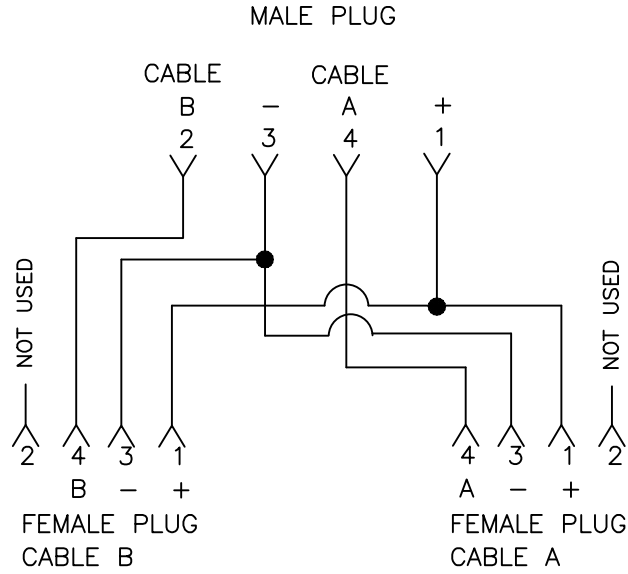
WIRING SCHEMATIC
