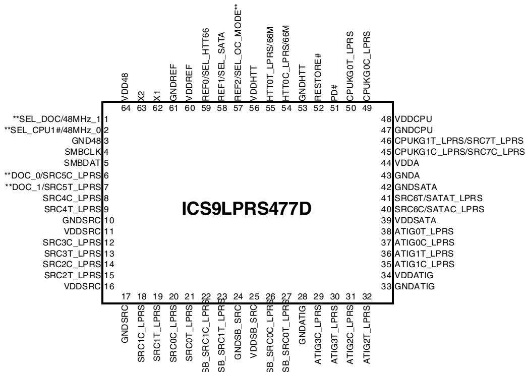
64-Pin MLF
