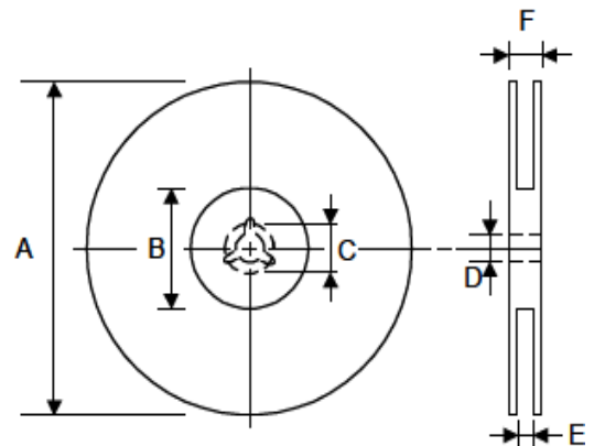
Reel Dimensions
