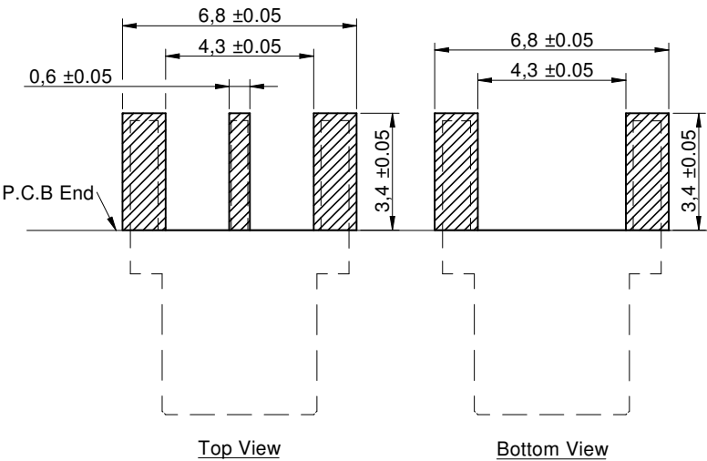
P.C.B Thickness: 1,1 mm
