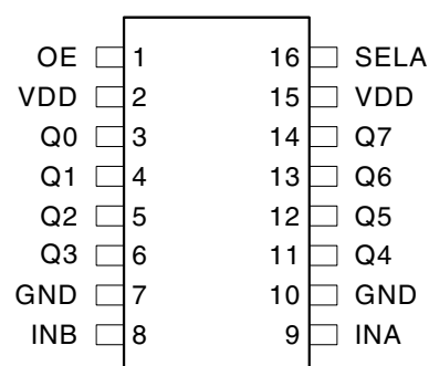
16 Pin TSSOP
