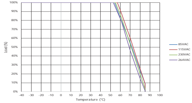
BAC05S12DC
