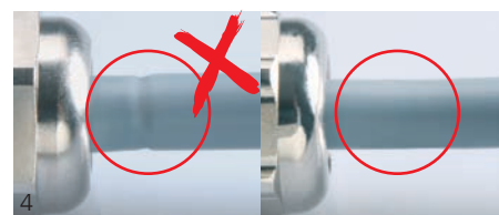
Einschnürung Constriction
