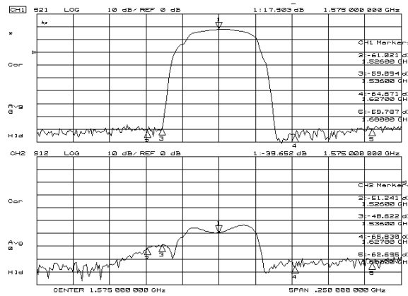
S21, S12
