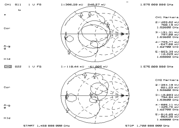
Zin, Zout
