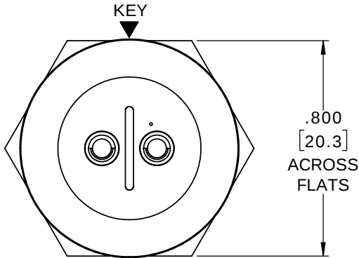
WIRING END W7382-2PG-P-300 SHOWN
