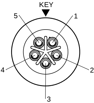
WIRING END W7382-5PG-P-300
