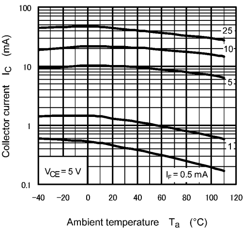
Fig. 11.13 I_C - T_a
