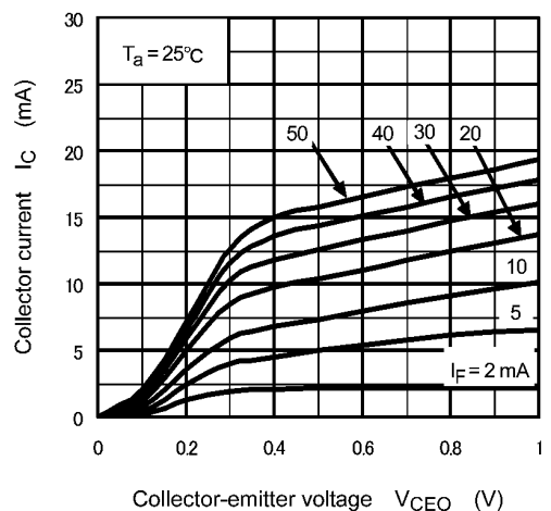
Fig. 11.8 I_C - V_{CE0}
