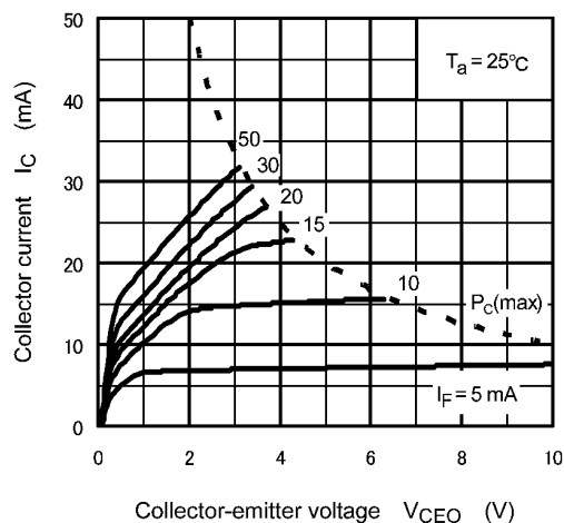
Fig. 11.7 I_C - V_{CE0}
