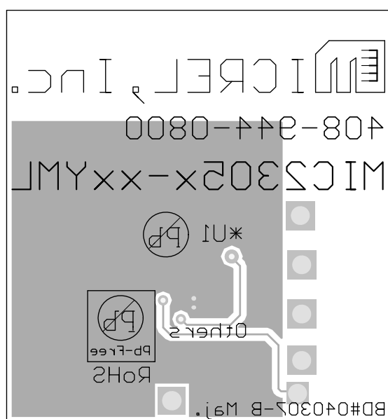
Bottom Layer
