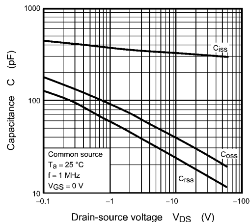
Fig. 8.8 C - V_{DS}
