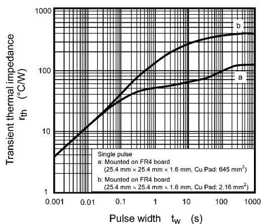
Fig. 8.11 r_{th} - t_w
