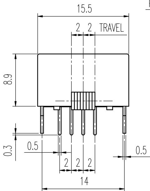
K DETAIL 2 : 1
