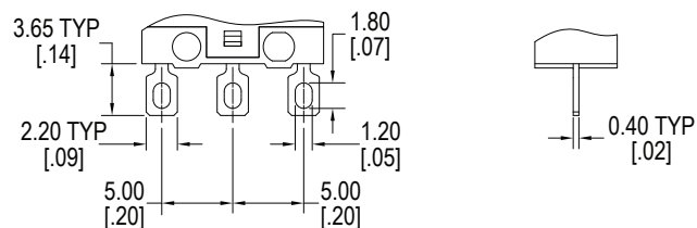
Solder Lug
