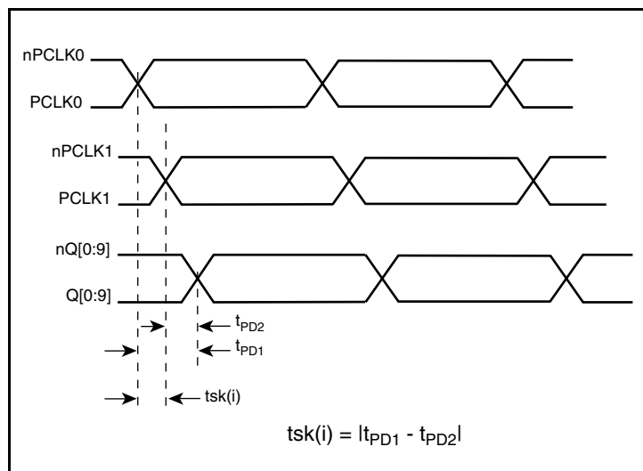
Input Skew
