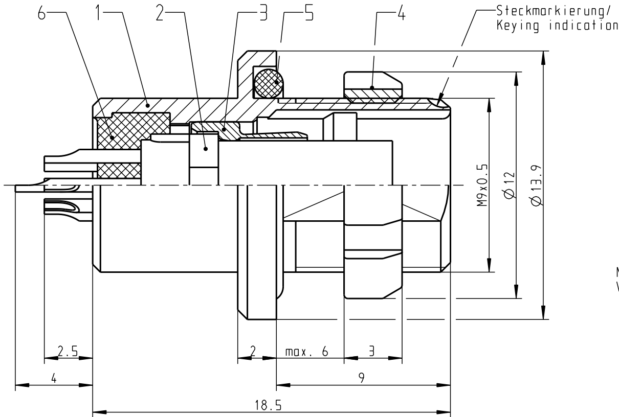
Nur Einsatz dargestellt/ View only insert
