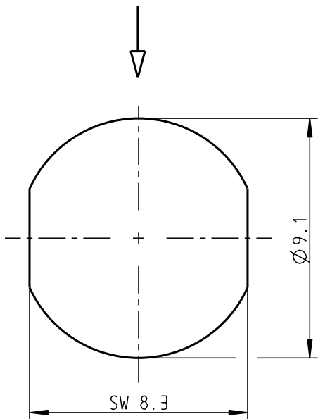
Steckmarkierung/ Keying indication
