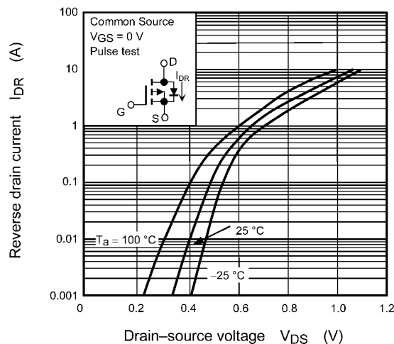
Fig. 8.9 I_{DR} - V_{DS}
