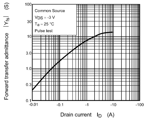
Fig. 8.8 |Y_{fs}| - I_D
