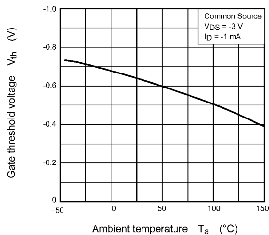
Fig. 8.7 V_{th} - T_a
