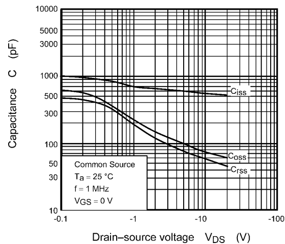
Fig. 8.10 C - V_{DS}
