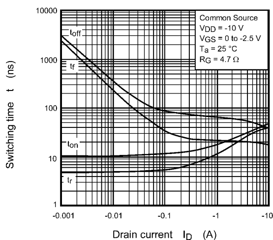
Fig. 8.11 t - I_D
