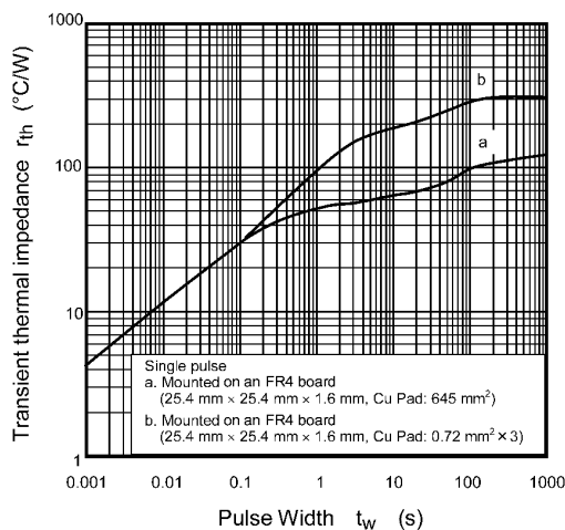
Fig. 8.13 r_{th} - t_w
