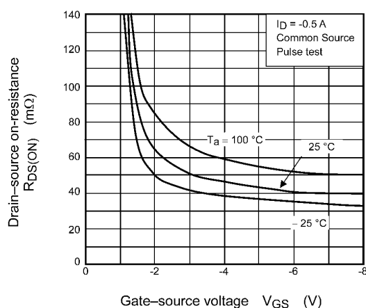
Fig. 8.3 R_{DS(ON)} - V_{GS}
