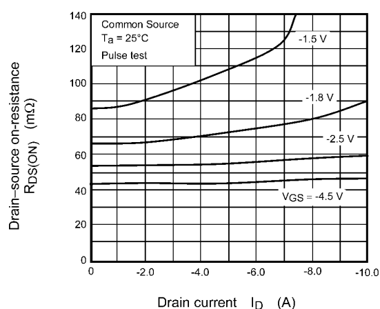
Fig. 8.5 R_{DS(ON)} - I_D
