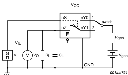
a. Test circuit
