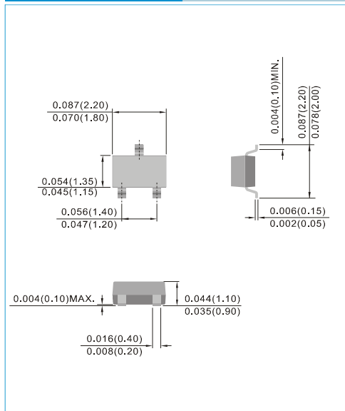
SOT-323 Unit : inch(mm)
