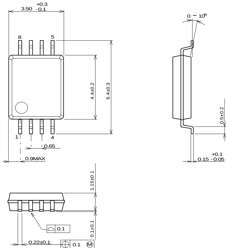
SSOP8 Package
