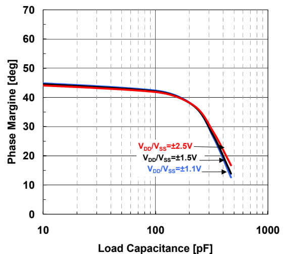
Phase Margin vs. Load Capacitance G_V=40dB , R_F=100k\Omega , R_G=1k\Omega , R_L=10k\Omega , V_{IN}=-30dBm , T_a=+25^\circ C
