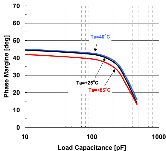
Phase Margin vs. Load Capacitance G_V=40dB , R_F=100k\Omega , R_G=1k\Omega , R_L=10k\Omega , V_{IN}=-30dBm , V_{DD}/V_{SS}=\pm 1.5V
